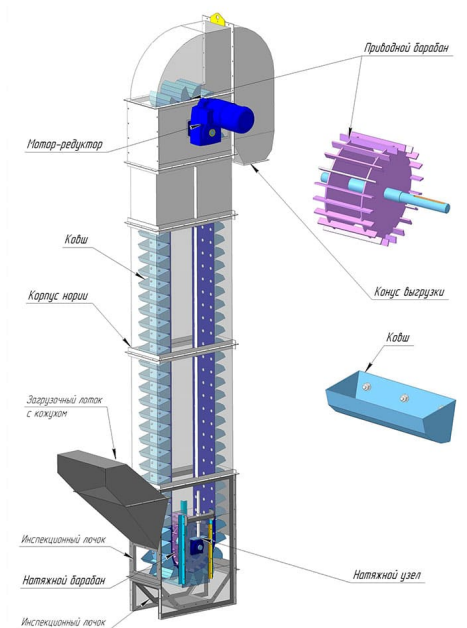
Схематическое изображение ковшового элеватора (нории)
